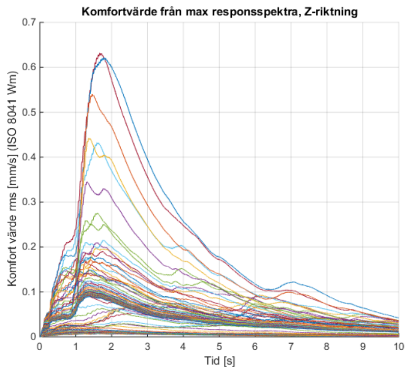
Figur 5.8 och 5.9. Resultat av responsspektraberäkningar för MP2_1 presenteras överst som maximalt komfortvärde för varje frekvens för de olika riktningarna och i tillhörande undre figur som funktion av tid (horisontellt tvärs spår) där varje plottad resultatlinje motsvarar en frekvenslinje.
