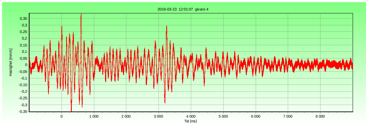
Bild 1. Kurvförlopp för högsta komfort dagtid 06-22, 2018-03-23 12:01:07.
