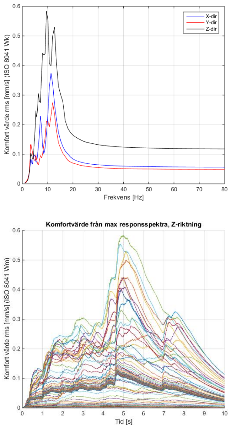
Figur 5.2 och 5.3. Resultat av responsspektraberäkningar för MP1_1 presenteras överst som maximalt komfortvärde för varje frekvens för de olika riktningarna och i tillhörande undre figur som funktion av tid (vertikalt) där varje plottad resultatlinje motsvarar en frekvenslinje.
