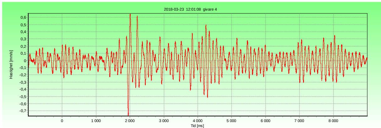
Bild 1. Kurvförlopp för högsta komfort gällande dagtid 06-22, 2018-03-23 12:01:08.
