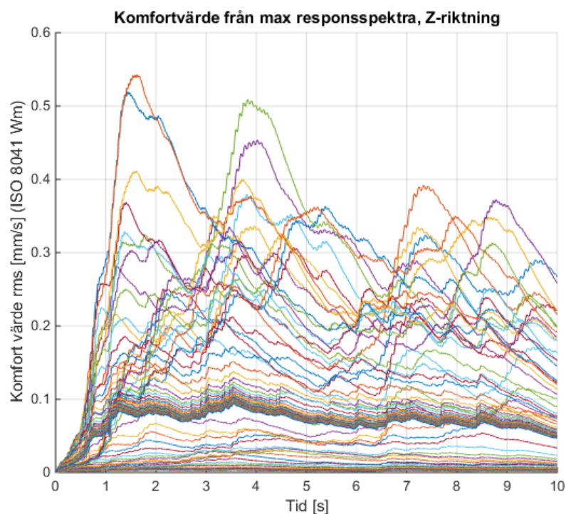
Figur 5.4 och 5.5. Resultat av responsspektraberäkningar för MP1_2 presenteras överst som maximalt komfortvärde för varje frekvens för de olika riktningarna och i tillhörande undre figur som funktion av tid (horisontellt tvärs spår) där varje plottad resultatlinje motsvarar en frekvenslinje.
