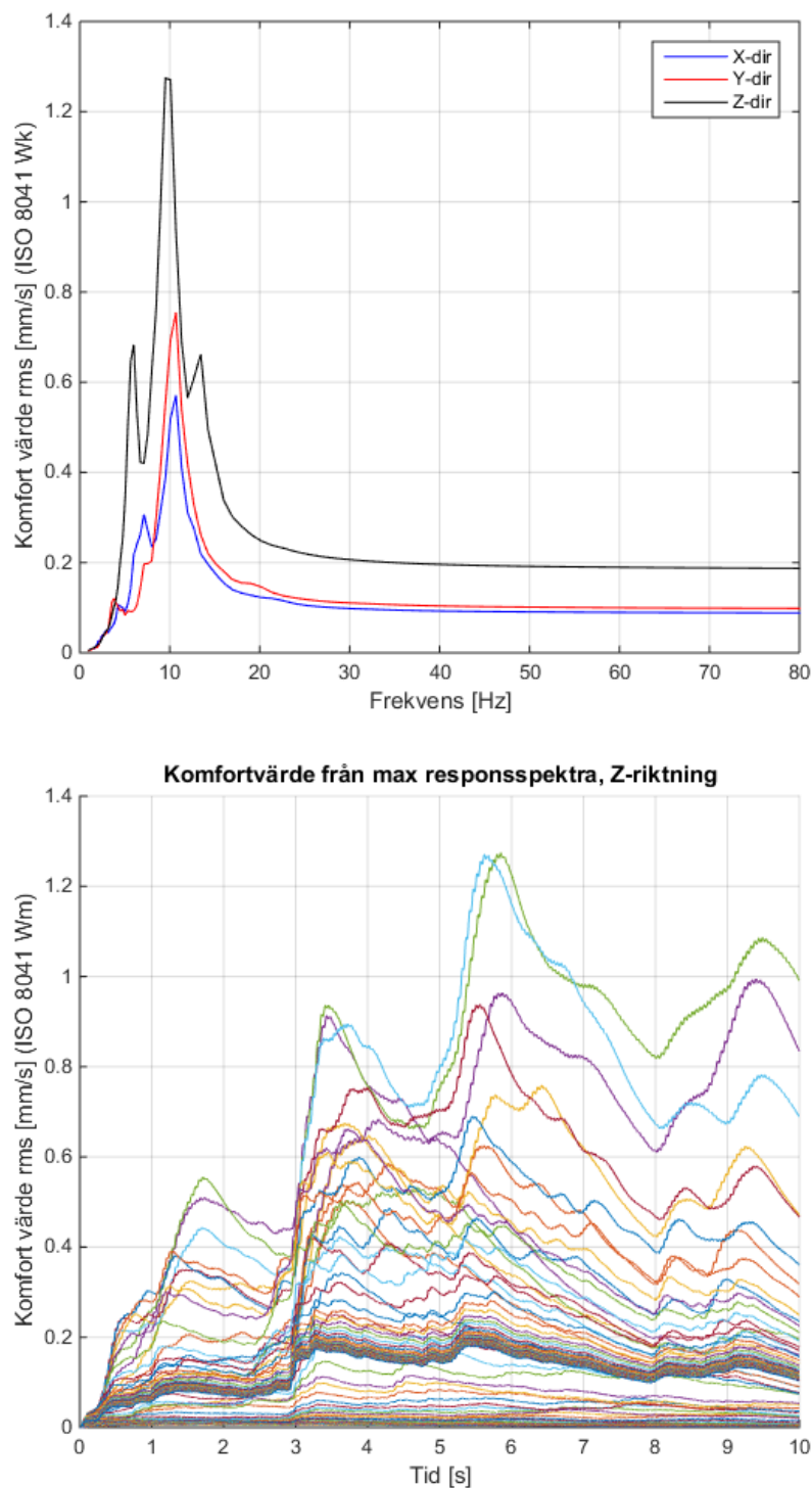
Figur 5.6 och 5.7. Resultat av responspektraberäkningar för MP1_3 presenteras överst som maximalt komfortvärde för varje frekvens för de olika riktningarna och i tillhörande undre figur som funktion av tid (horisontellt tvärs spår) där varje plottad resultatlinje motsvarar en frekvenslinje.
