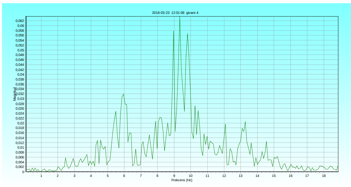
Bild 2. Frekvensspektrum för kurvförlopp bild 3.
